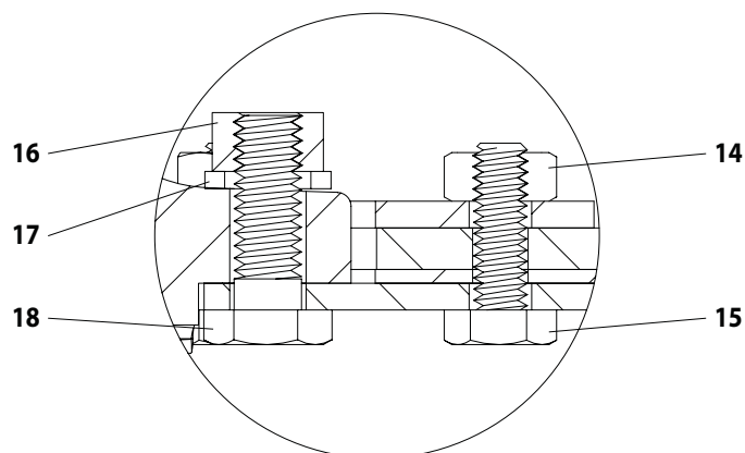
视图 "B"
